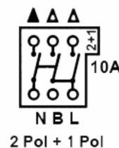
Koblingskjema
