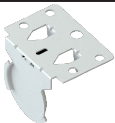
Stenderfeste for R-line stenderskrue med spiker Tilpasset boks serie R-line 60 - 72 - 80 - 92 - 120
