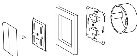
Montering utenpå veggboксer med skruer.
